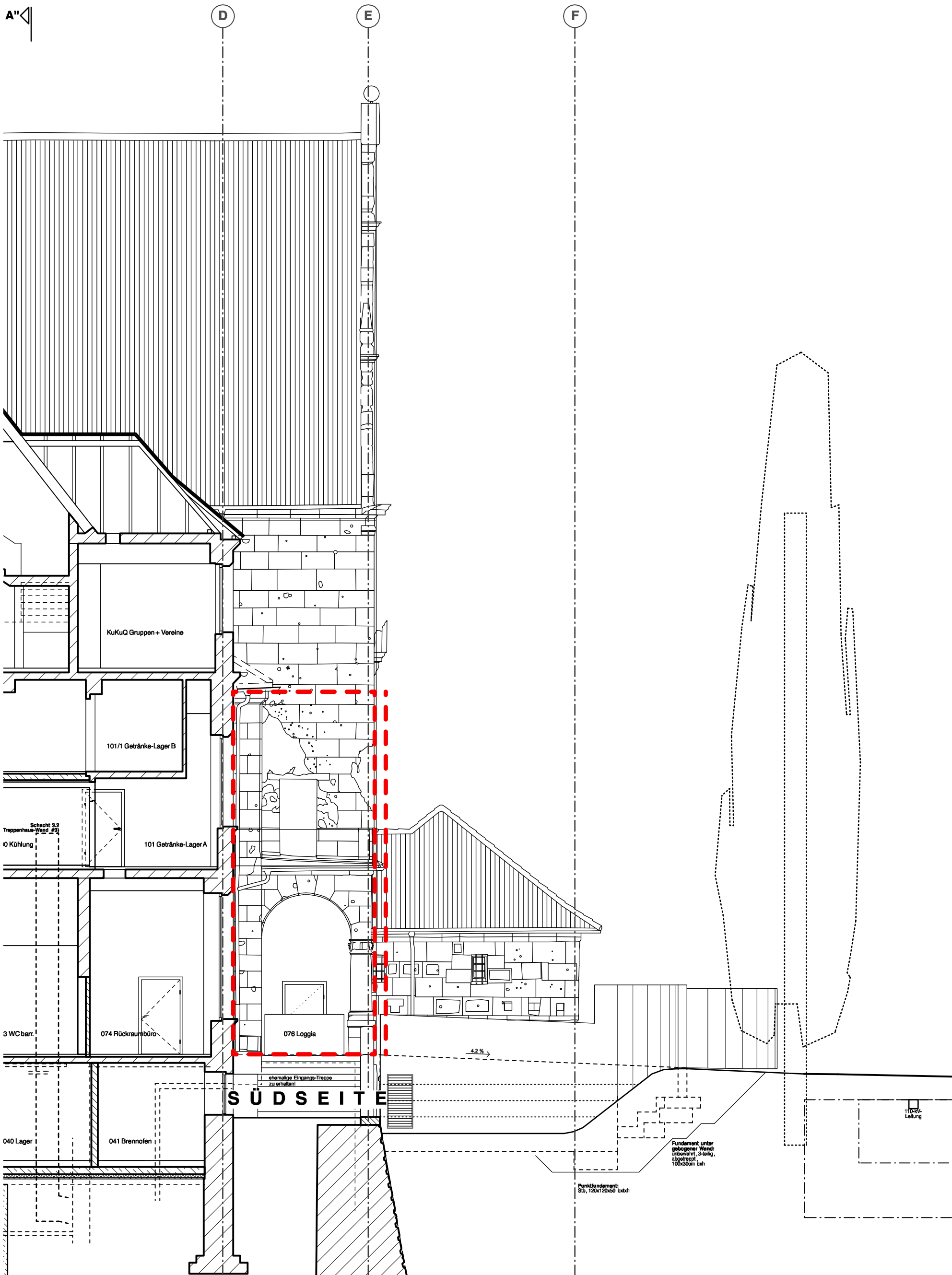
GENERALSANIERUNG KÜNSTLERHAUS NÜRNBERG 3.BA / FLORIAN NAGLER ARCHITEKTEN GmbH / AUSSCHNITT SCHNITT H-H / M 1:100
